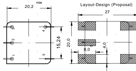
QO2024S SMD-Version
